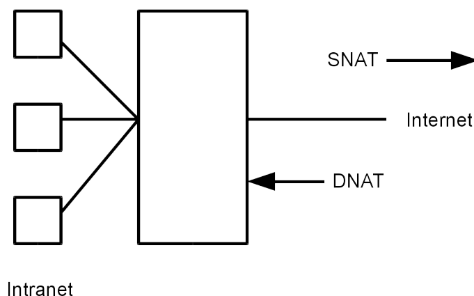
Рис. 9.1: Механизм NAT
