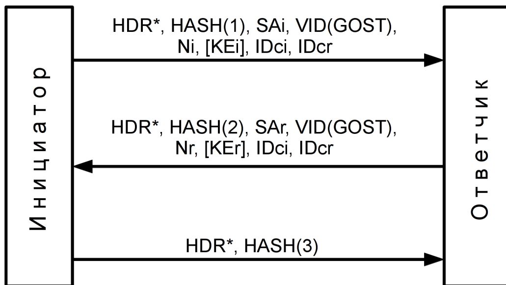
Рис. 41.3: Фаза 2
