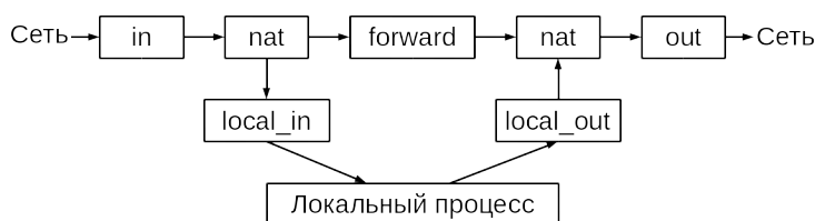
Рис. 7.1: Фильтрация
