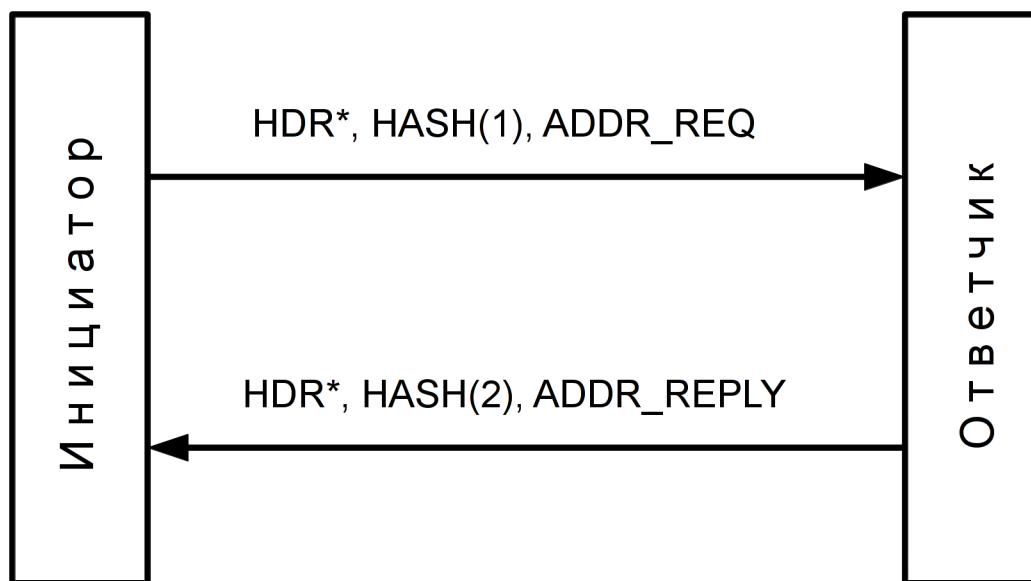
Рис. 41.4: Фаза ModeConfig
