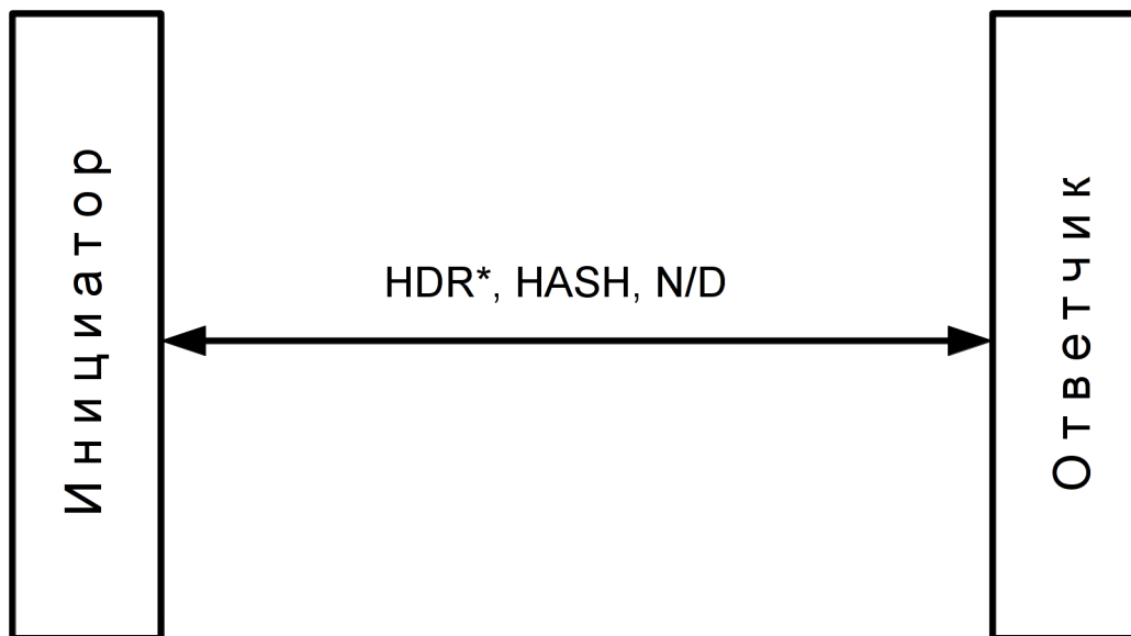
Рис. 41.5: Сообщения уведомлений
