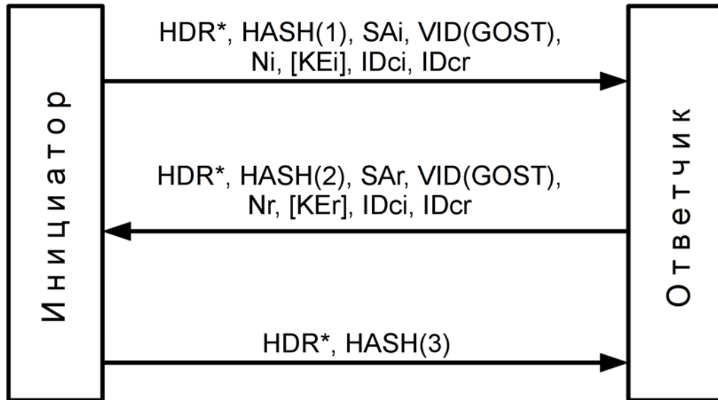
Рис. 52.3: Фаза 2
