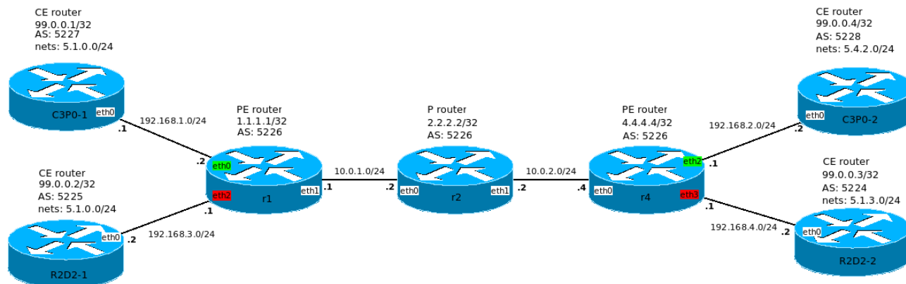
Рис. 51.2: Схема 2: MPLS-L3VPN
