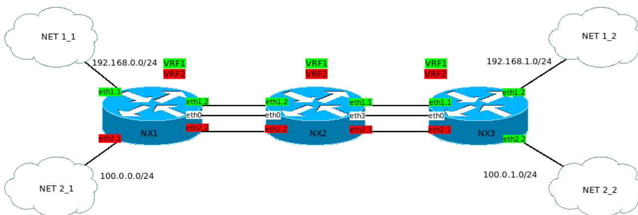
Рис. 51.1: Схема 1: vrf-lite + OSPF
