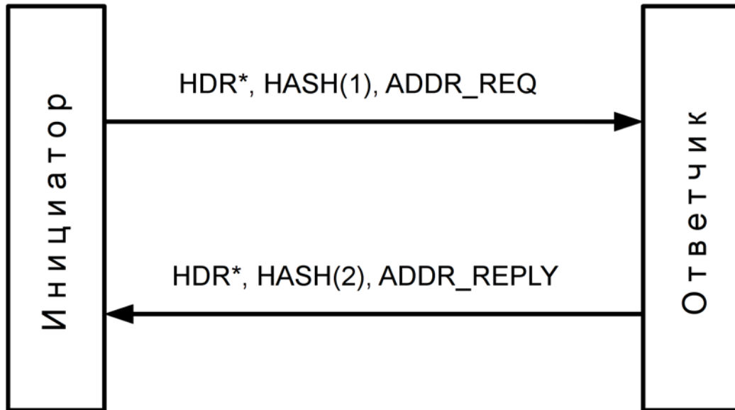
Рис. 52.4: Фаза ModeConfig
