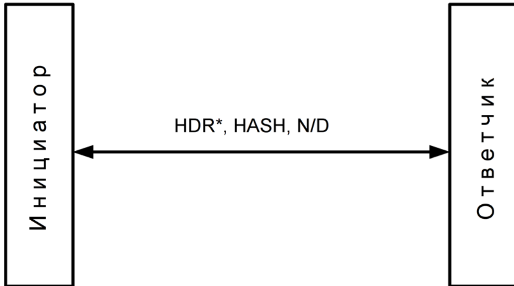
Рис. 52.5: Сообщения уведомлений
